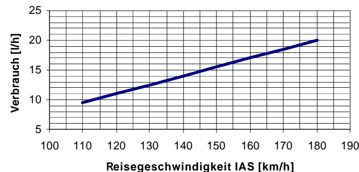
Kraftstoffverbrauch bei max. Abflugmasse
